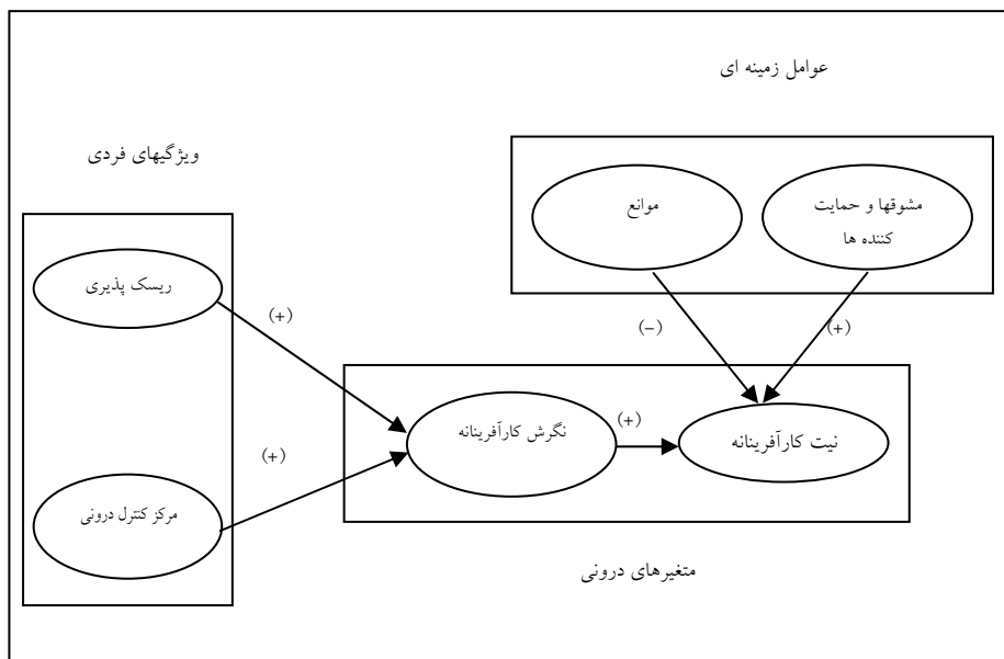
شکل ۴ - مدل ساختاری قصد کارآفرینانه
